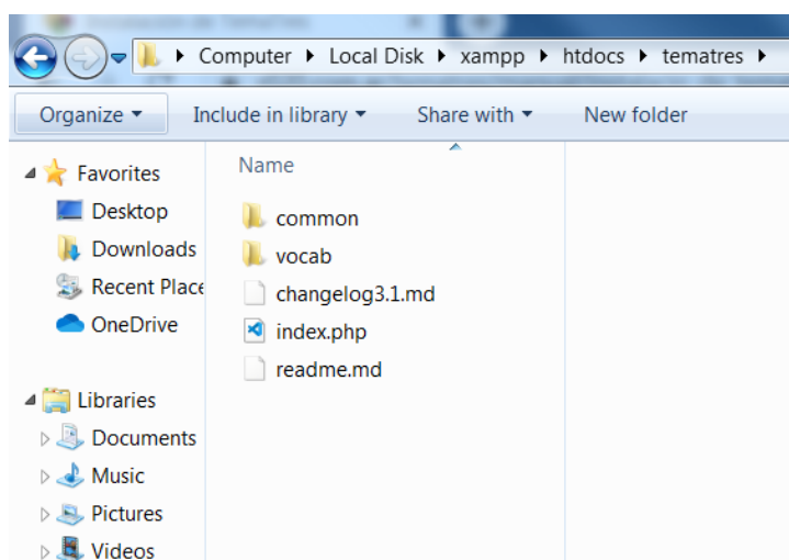
Figura 11: ruta TemaTres
