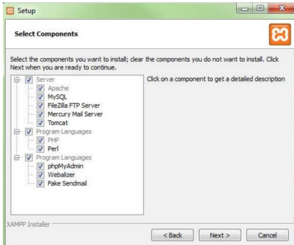
Figura 9: Setup XAMPP
