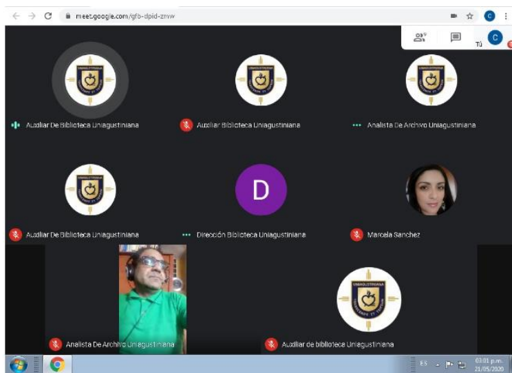
Figura 14: Entrega Microtesauro.
